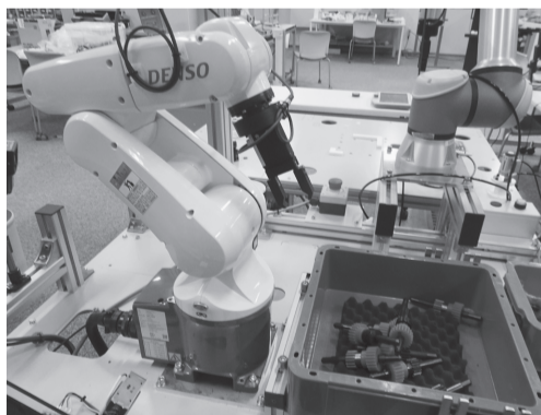
重なる製品を仕分けるロボット
